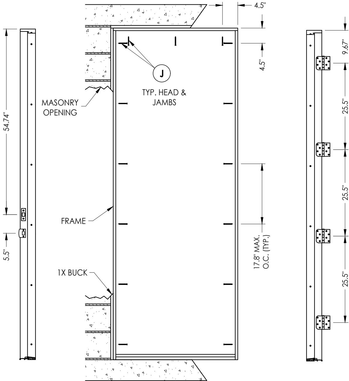
STRIKE JAMB
