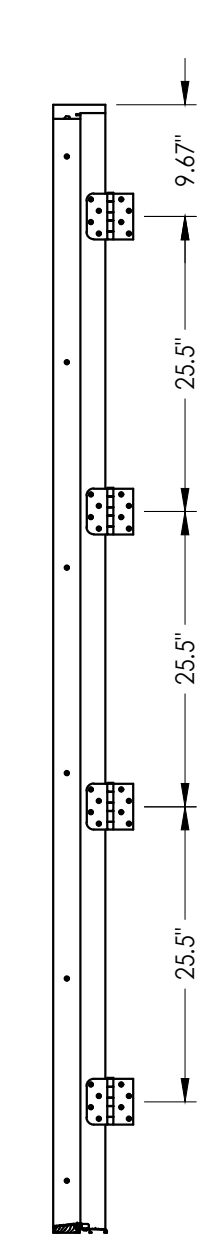
HINGE JAMB
